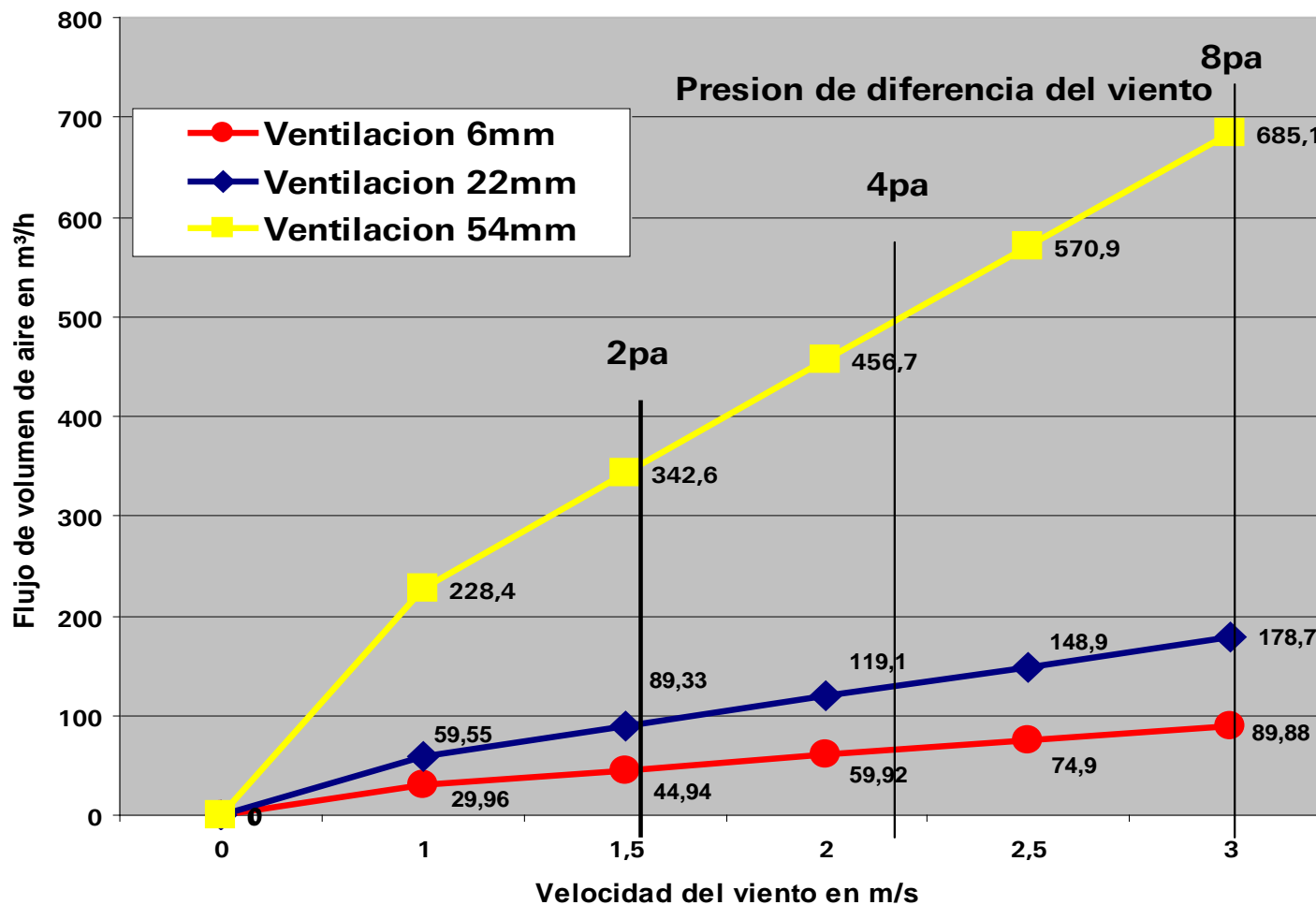
Flujo de aire dependiendo de la velocidad del viento
