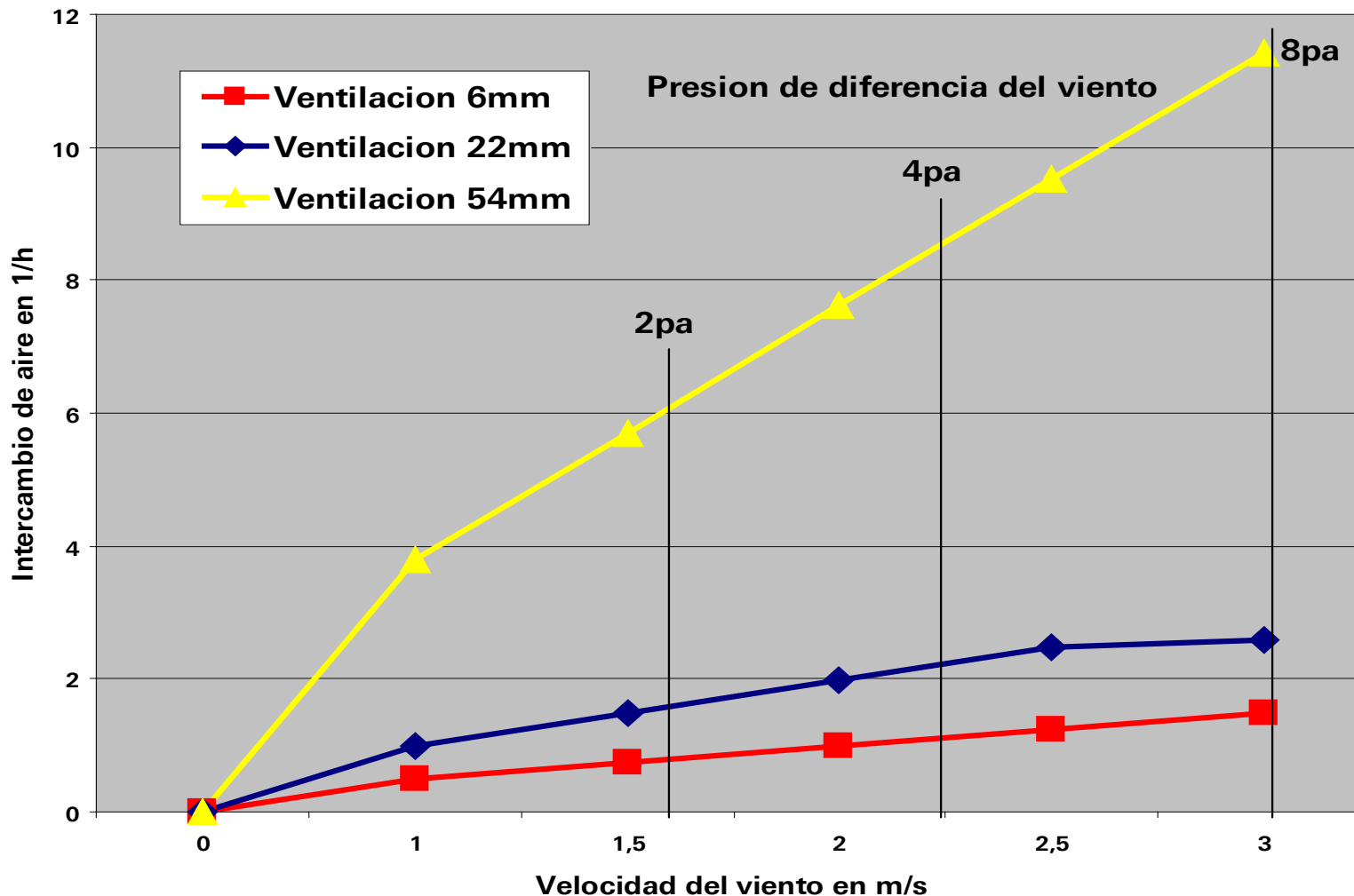
Intercambio de aire dependiendo de la velocidad del viento
