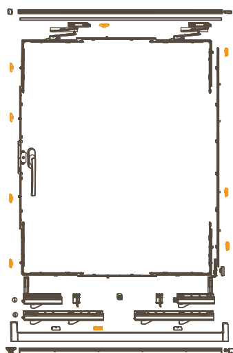
Herraje Oscilobatiente Seguridad básica 1 hoja
