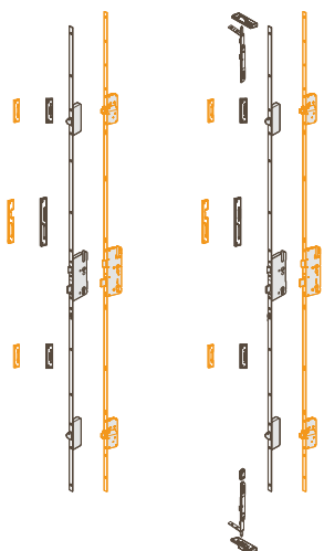
Herrajes para puerta de calle
