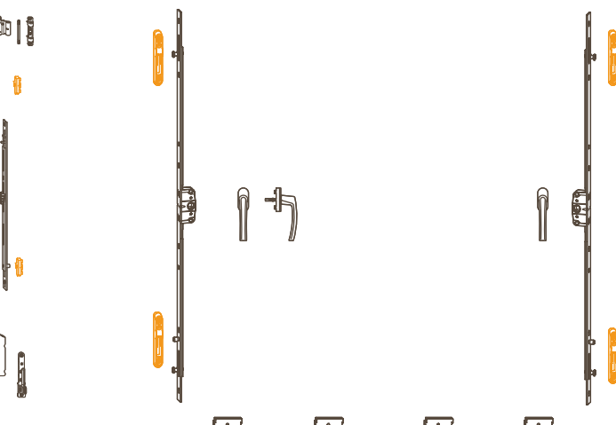
Herraje 2 hojas para corredera lineal
